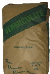
VERMICULITE
